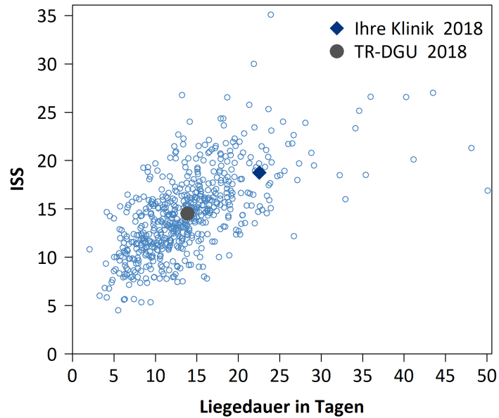
Abbildung 24: Korrelation zwischen Liegedauer und Verletzungsschwere über alle Kliniken in 2018
