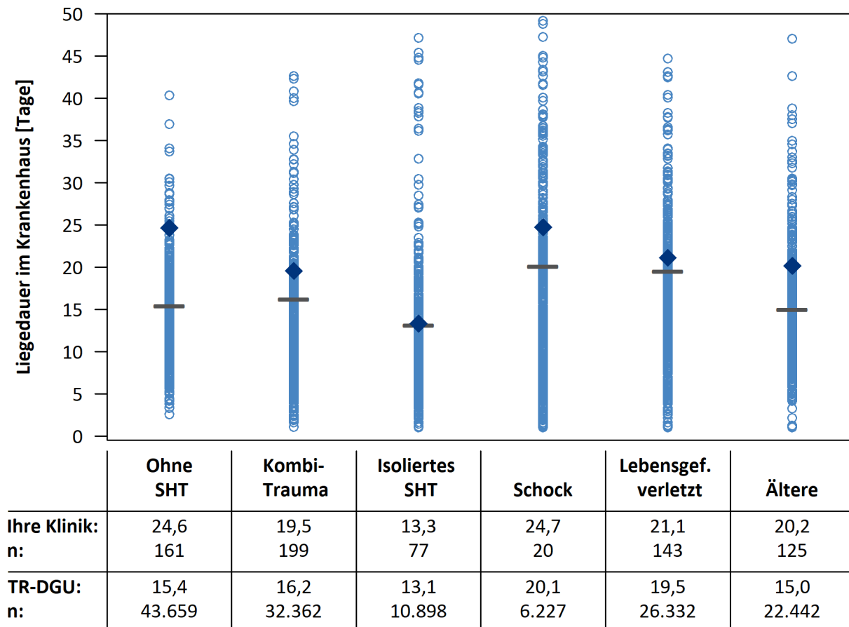
Abbildung 27: Liegedauer [Tage] und Patientenzahlen im Krankenhaus getrennt nach Subgruppen, Definition siehe Tab. 14, Patienten 2016-2018, Ihre Klinik, — TR-DGU, o einzelner Klinikwert
