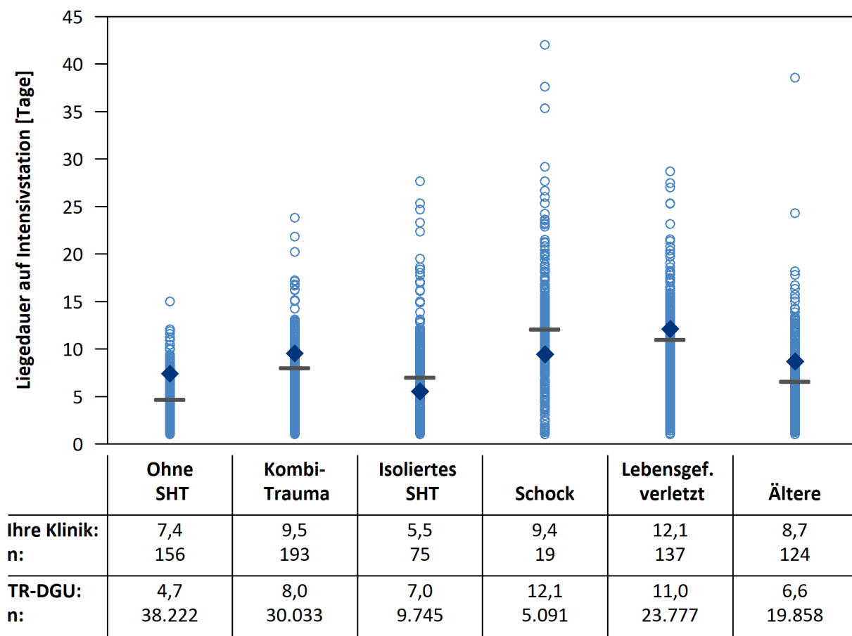
Abbildung 26: Liegedauer auf Intensivstation [Tage] und Patientenzahlen getrennt nach Subgruppen, Definition siehe Tab. 14, Patienten 2016-2018, Ihre Klinik, — TR-DGU, o einzelner Klinikwert
