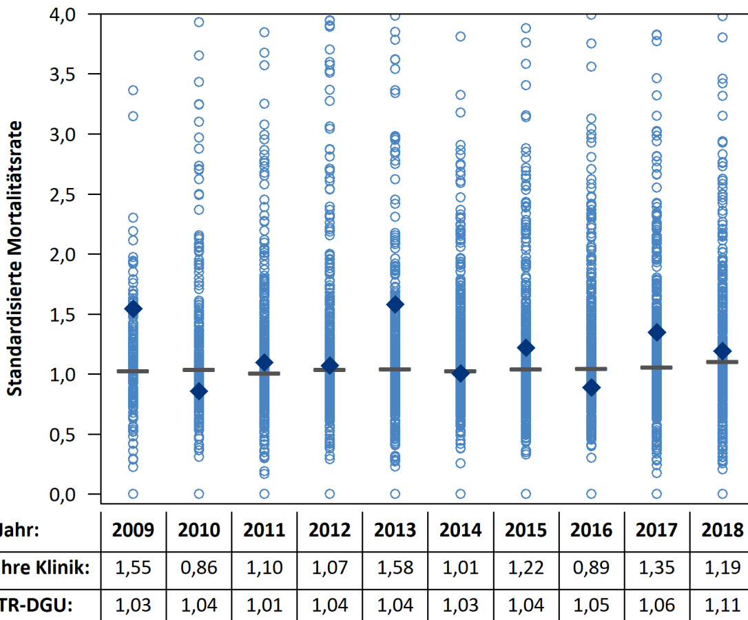
Abbildung 23: Standardisierte Mortalitätsratio von Ihrer Klinik und vom — TR-DGU im Vergleich zu den einzelnen Klinikwerten im TR-DGU für die Jahre 2009-2018
