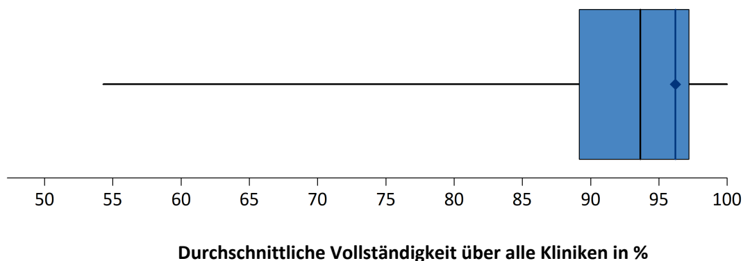
Abbildung 28: Verteilung der Vollständigkeitsrate der Daten aus 2018 über alle Kliniken und Vollständigkeitsrate Ihrer Klinik
