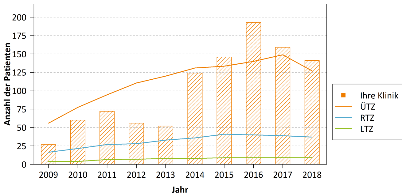
Abbildung 19: Fallzahlen Ihrer Klinik im Basiskollektiv des TR-DGU von 2009 - 2018 (Balken) sowie die mediane jährliche Fallzahl pro Traumastufe (Kurven). Farbe der Balken = aktuelle Traumastufe Ihrer Klinik (Überregionales Traumazentrum, ÜTZ)
