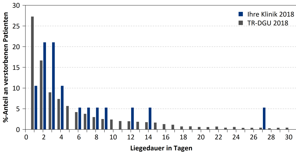
Abbildung 25: Versterbenszeitpunkt der Patienten Ihrer Klinik [Liegedauer in Tagen] im Vergleich zum TR-DGU in 2018
