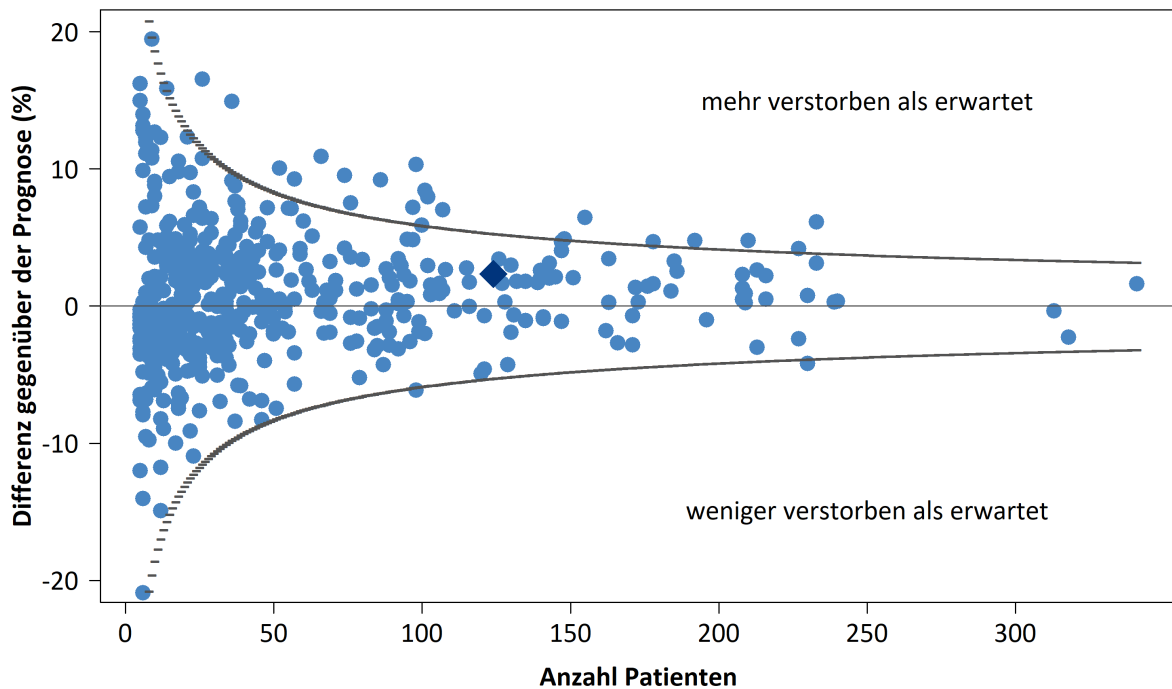
Abbildung 3: Differenz zwischen Letalität und Letalitätsprognose (RISC II) aller am TR-DGU teilnehmenden Kliniken mit mehr als 5 Fällen für das Jahr 2018, : Ihre Klinik
